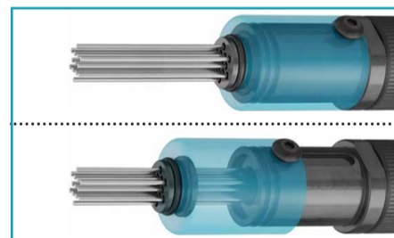
Justerbart nålbrett med integrert nålføring sikrer lang brukstid
