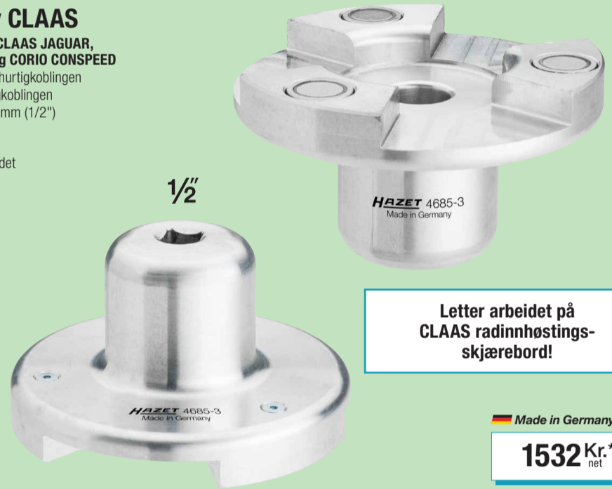
Betjening ved hjelp av en skralle gjennom en innsatt 12,5 mm (1/2") firkantholder
